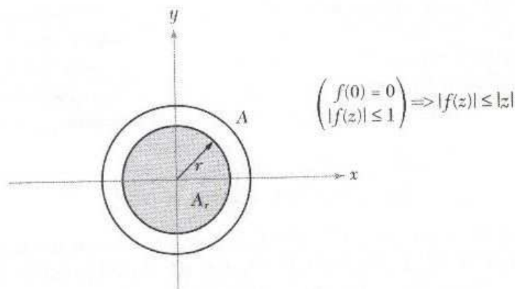
Figure 2.5.2: Schwarz Lemma
